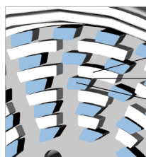
Fristam FSP lid Shearing clearance 0,5 mm Fristam FSP impeller
